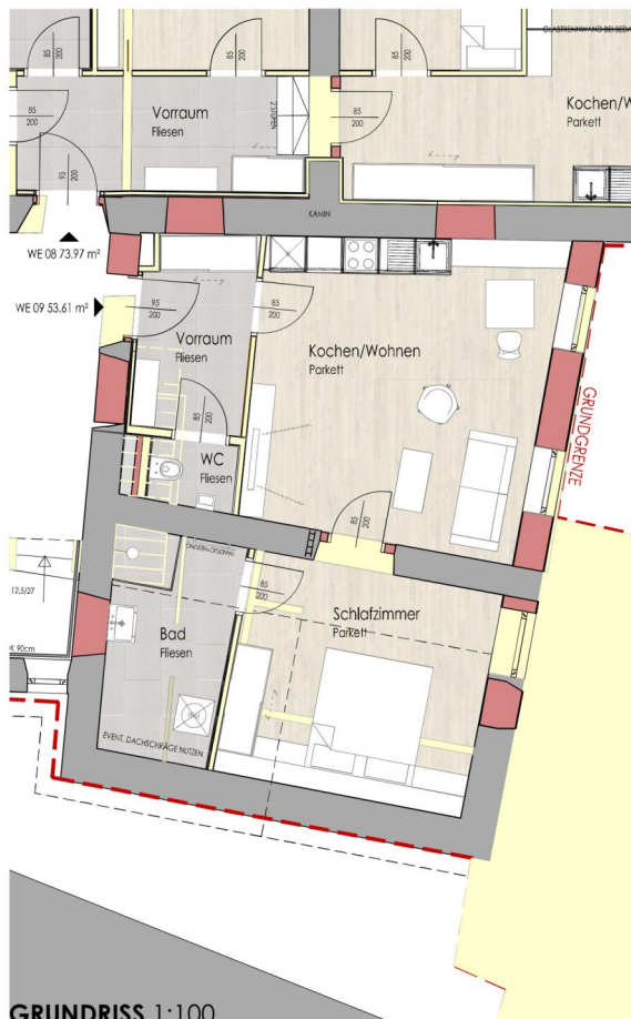
GRUNDRISS 1:100
